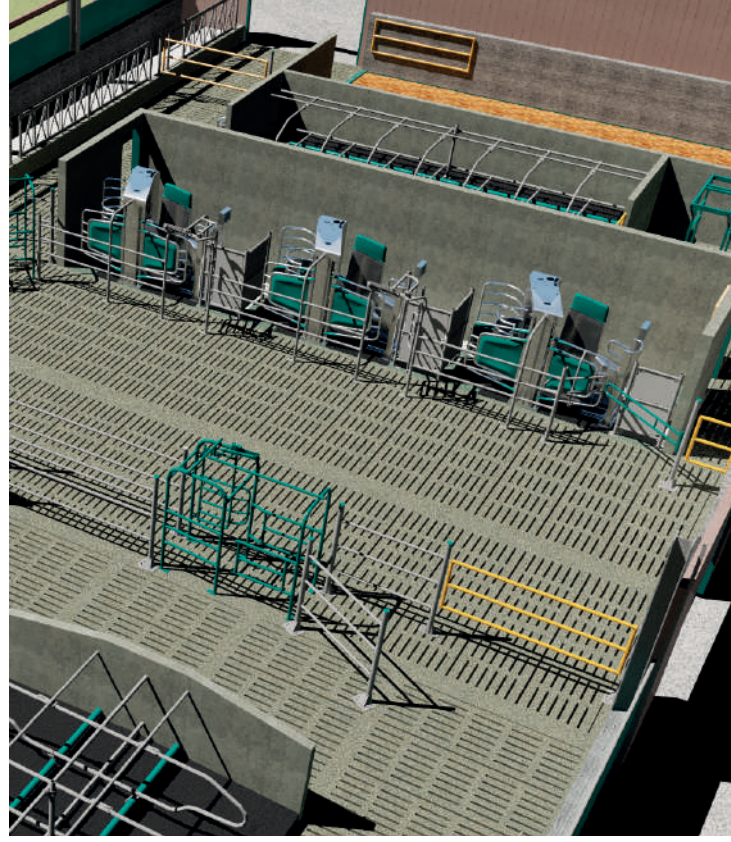
Ayırıcı kapılı Multi-box kurulumu
