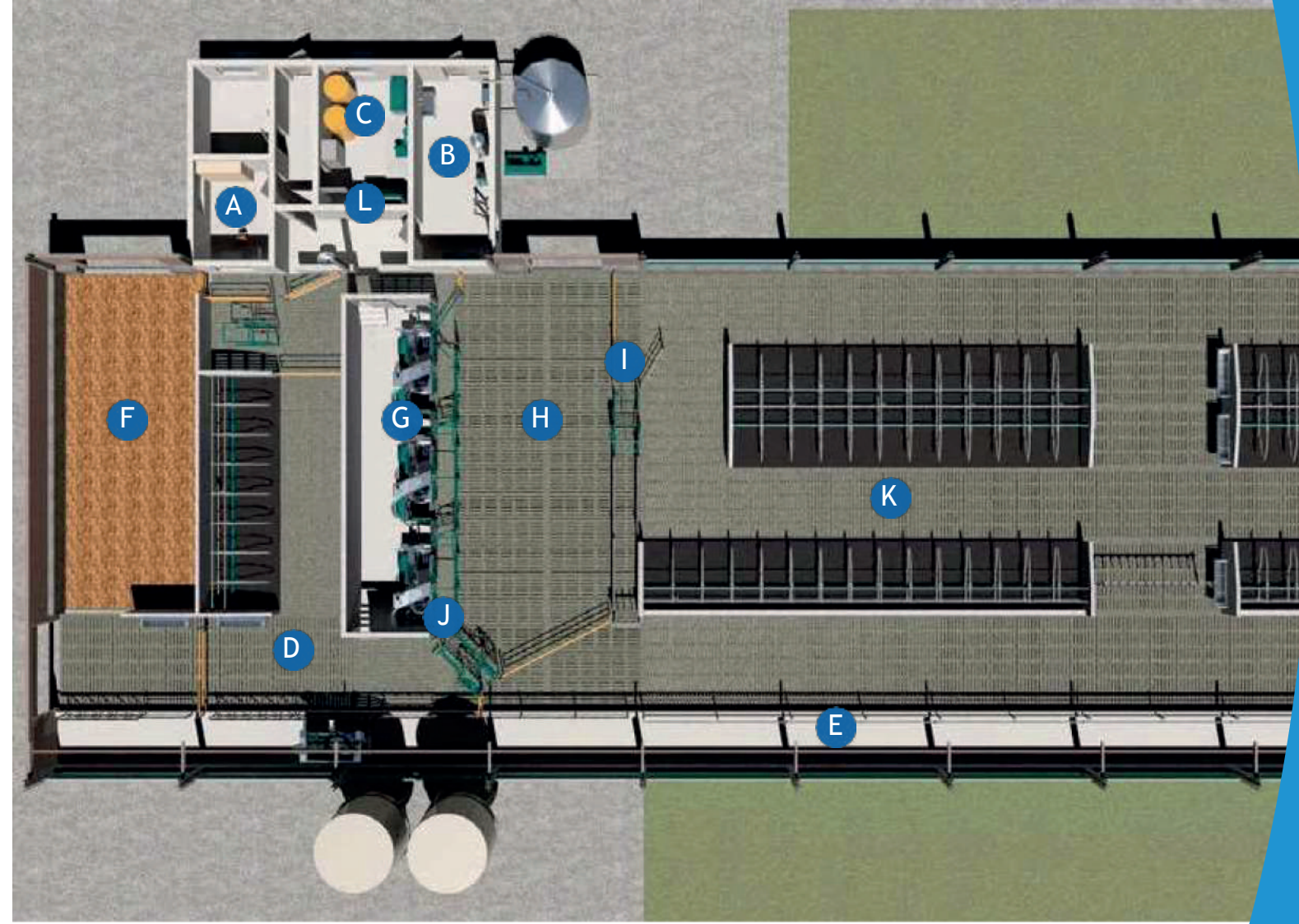
Ayırıcı kapılı Multi-box kurulumu
